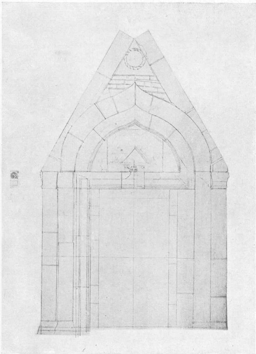
Чертеж современного состояния облицовки северного портала
