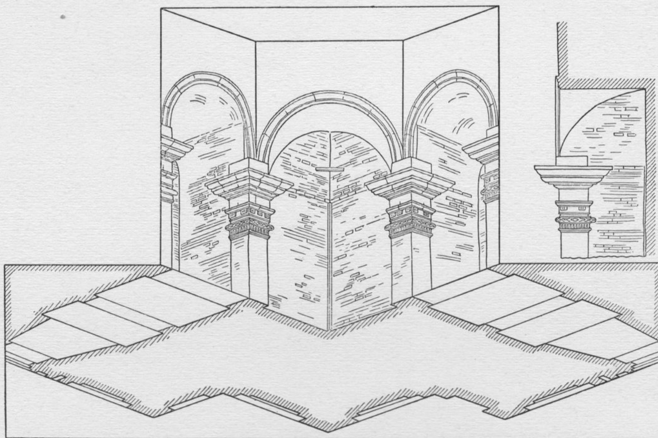
Аксонметрический рисунок угловых пилястров
