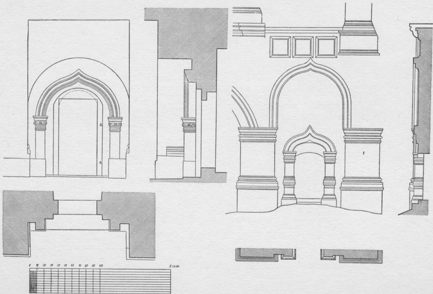
Слева — детали двери в подклет. Справа — детали северного крыльца
