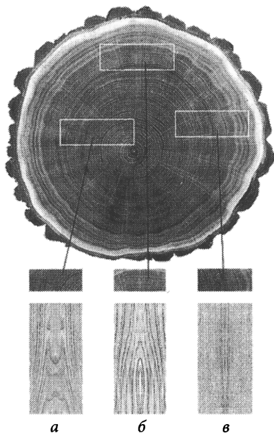
Рис. 92. Распил древесины:
