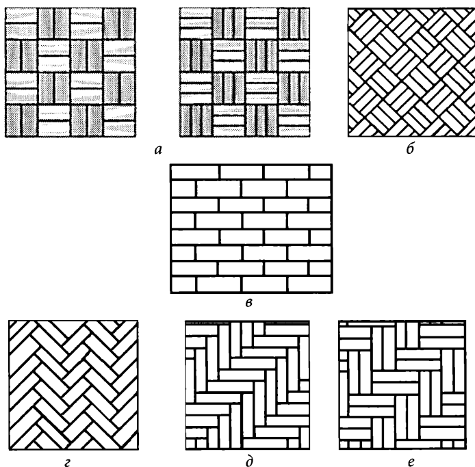
Рис. 87. Укладка паркета:
